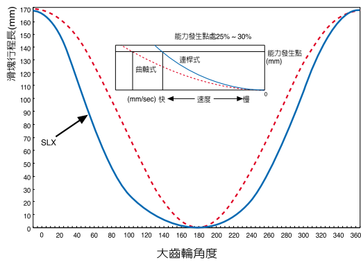
滑塊運動曲線(B-Type)
