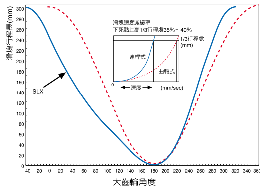
滑塊運動曲線(D-Type)
