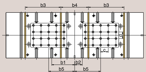
圖形四 (含舉模器用"U"型溝)
